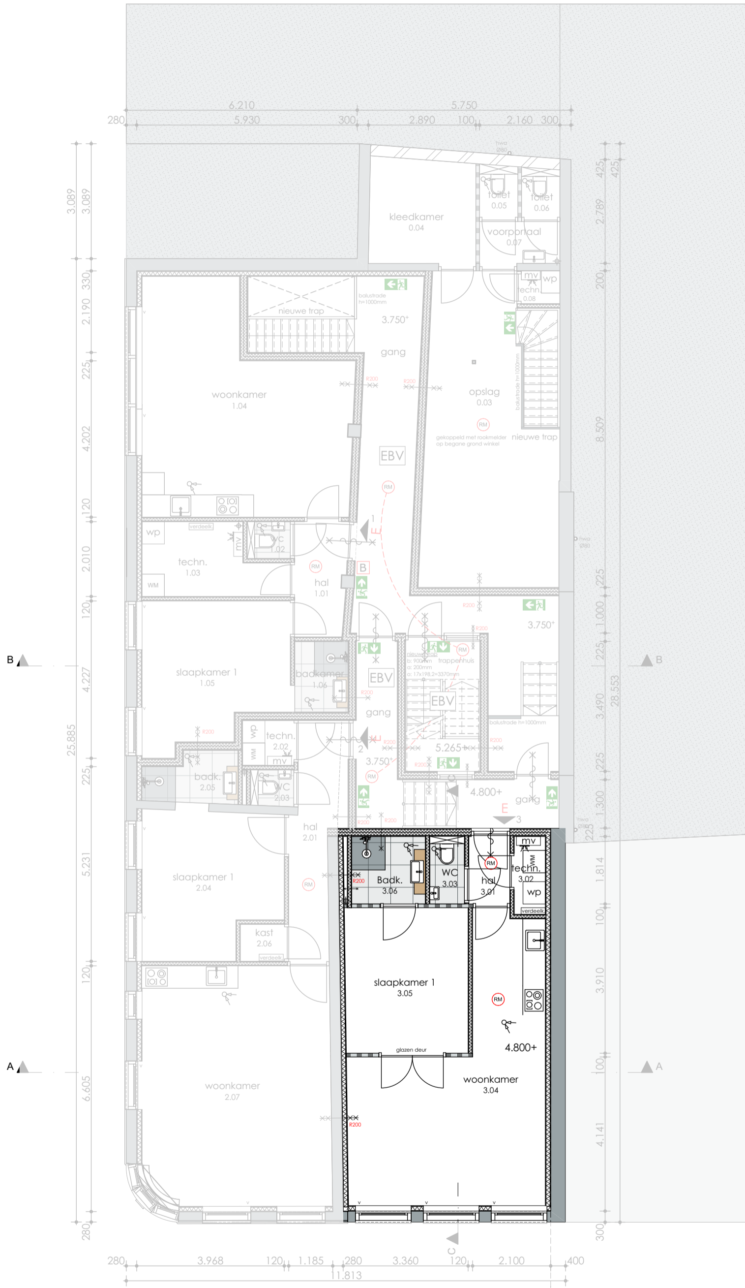
1e verdieping 3.750+
